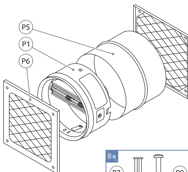
DN160 ... DN200
