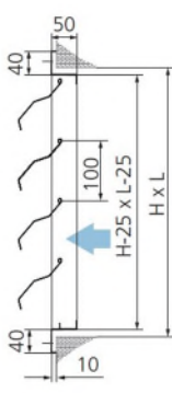
Tipo 1 con rete
