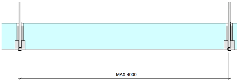
Con supporto per canale in acciaio
