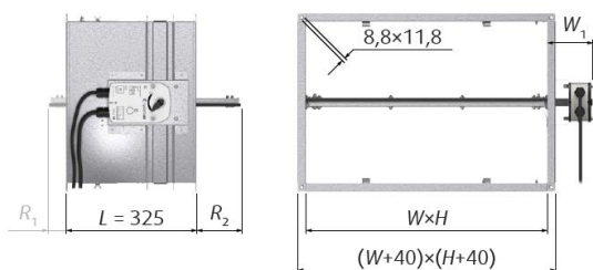
Figura 1 Dimensioni serranda rettangolare WxH = 200x200 mm fino a 1200x800 mm
