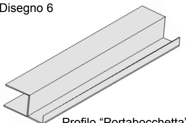
Profilo "Portabocchetta"
