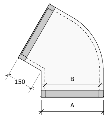
CURVA 60° DA _ _ _ 60
