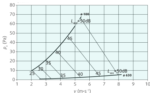
Perdite di carico e livello di potenza sonora serranda circolare
