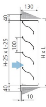
Tipo 2 con rete
