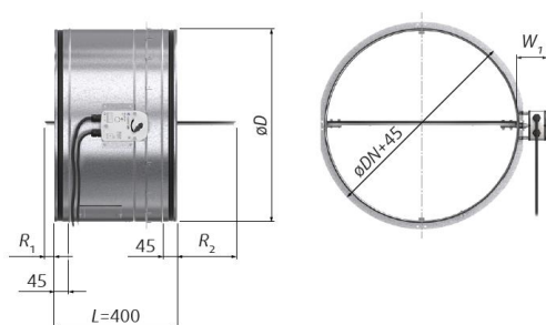
Figura 3 Dimensioni serranda circolare
