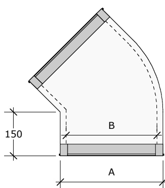
CURVA 45° DA _ _ _ 45
