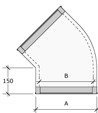
CURVA 45° DB _ _ 45
