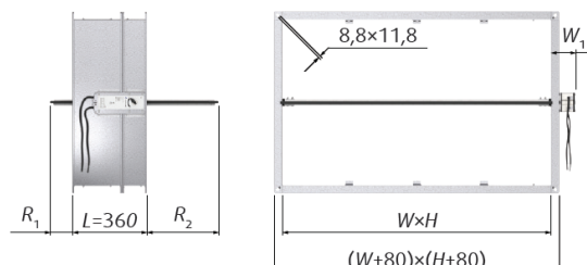
Figura 2 Dimensioni serranda rettangolare con W > 1200 mm fino a 1500x800 mm
