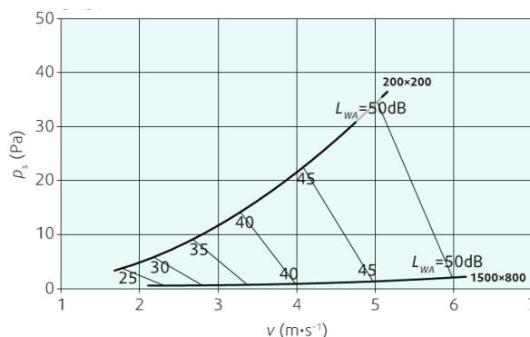
Perdite di carico e livello di potenza sonora serranda rettangolare
