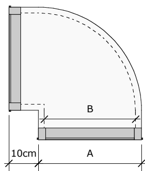
S1 CURVA 90° DA _ _ _ 90S1
