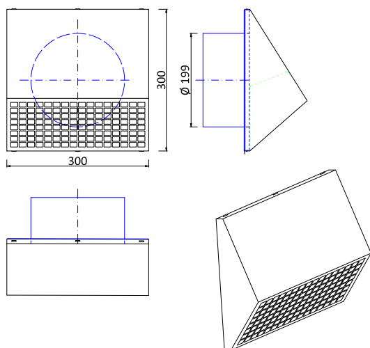
GRIGLIA ESTERNA cod. VMGAIR16200
