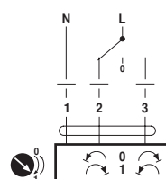
AC 230 V, 3-punti
