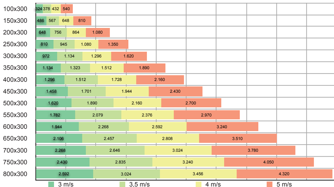
Altezza condotta h = 300 mm
