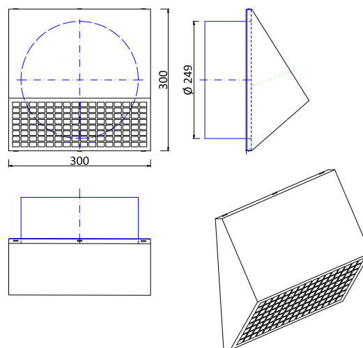
GRIGLIA ESTERNA cod. VMGAIR16250
