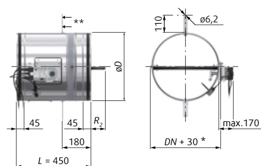
Fig. 5: Dimensioni della serranda tagliafuoco SFC 3G con servomotore - DN da Ø 100 a 630 mm
