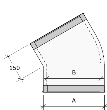
CURVA 30° DA ___ 30
