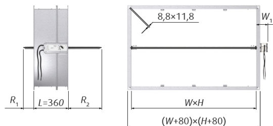
Figura 2 Dimensioni serranda rettangolare con W>1200 mm fino a 1500x800 mm
