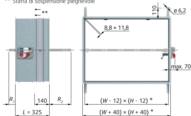
Fig. 8: Dimensioni della serranda tagliafuoco con attuatore manuale SFR-3G - dimensioni nominali da 100x100 mm a 1200x800 mm
