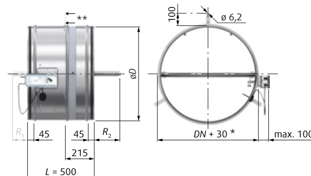
Fig. 7: Dimensioni della serranda tagliafuoco SFC 3G con servomotore - DN da Ø 710 a 1000 mm
