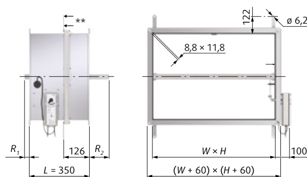
Fig. 11: Dimensioni della serranda tagliafuoco con servomotore SFR - dimensioni nominali da W > 1200 mm e/o H > 800 mm a 1600x1000 mm
