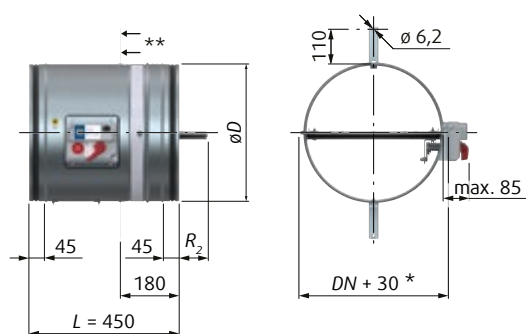
Fig. 4: Dimensioni della serranda tagliafuoco SFC 3G con attuatore manuale - DN da Ø 100 a 630 mm
