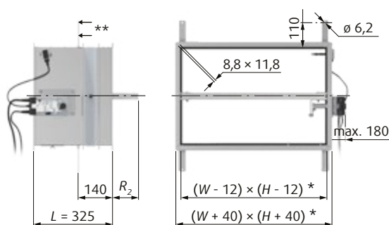
Fig. 9: Dimensioni della serranda tagliafuoco con servomotore SFR-3G - dimensioni nominali da 100x100 mm a 1200x800 mm
