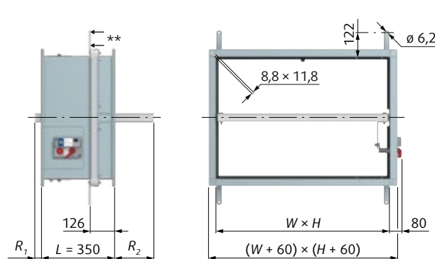
Fig. 10: Dimensioni della serranda tagliafuoco con attuatori manuale SFR - dimensioni nominali da W > 1200 mm e/o H > 800 mm a 1600x1000 mm
