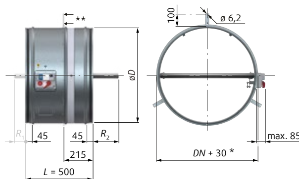
Fig. 6: Dimensioni della serranda tagliafuoco SFC 3G con attuatore manuale - DN da Ø 710 a 1000 mm
